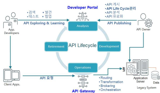
그림 3. API 라이프사이클과 관리 [5] Fig. 3. API life cycle management
